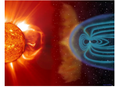
कोरोनल मास एजेक्सन
